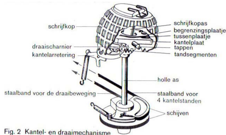
Fig. 2 Kantel- en draaimechanisme
