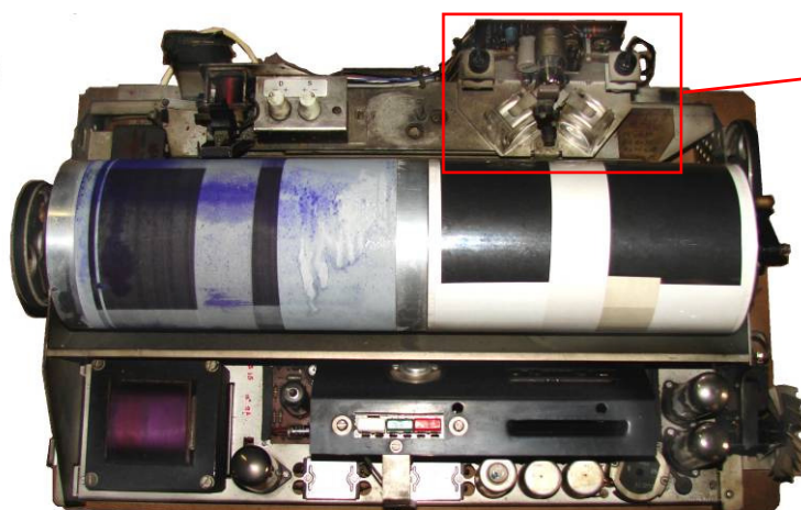
Links: schrijfkop (inbrandstift) op stencil, rechts leeskop
