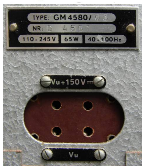
achterkant: kenplaatje en signaaluitgang
