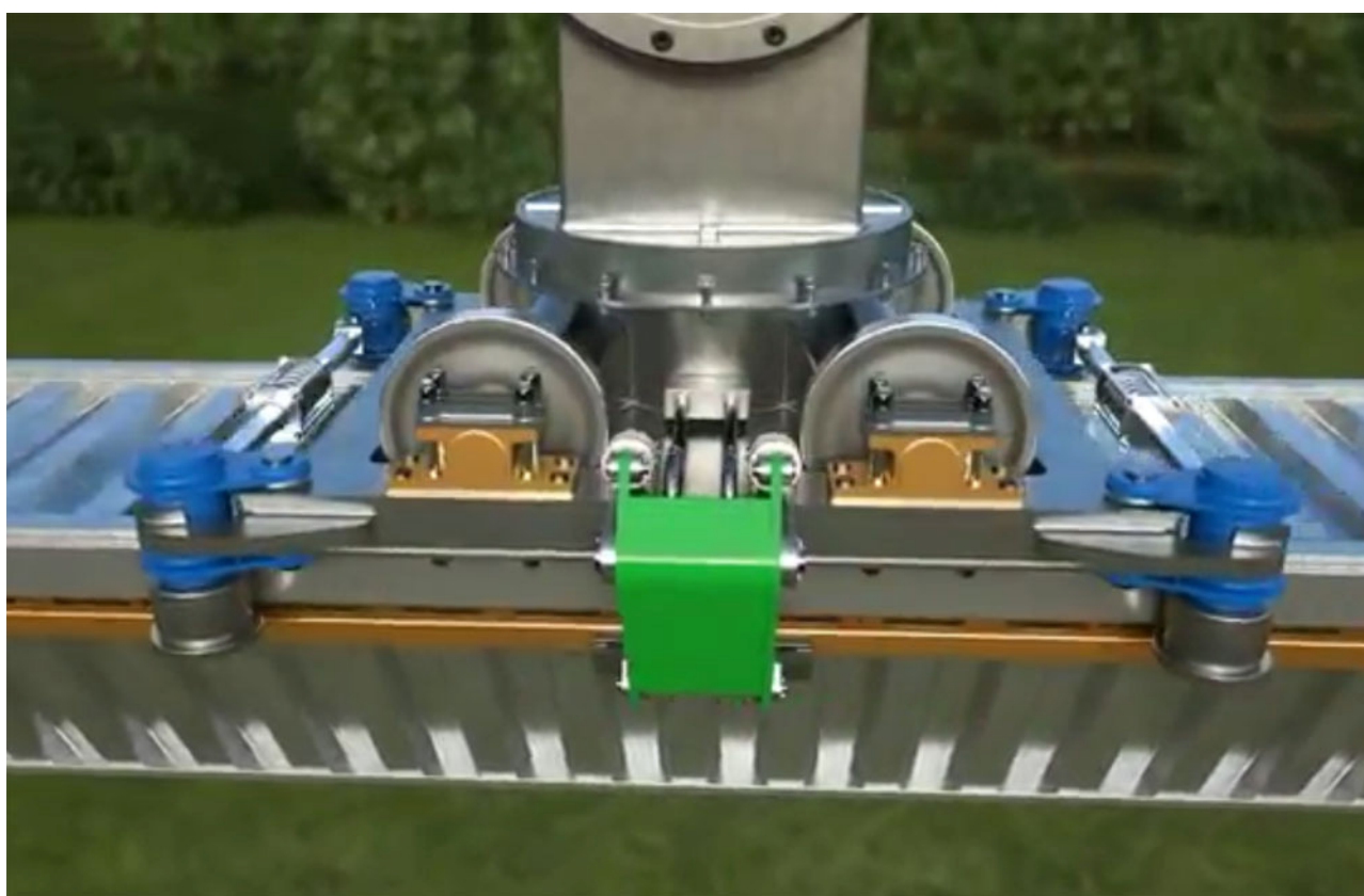
Foto 2 Volgwagentje met stroomafnemers
